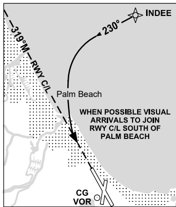
"RWY 14 VISUAL"
